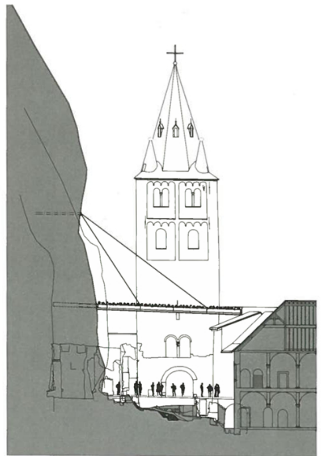
Secțiune transversală / Cross section
