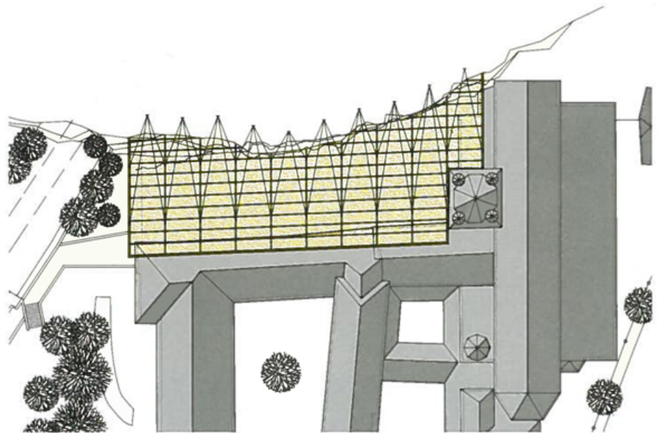
Vedere de sus / Roof plan
